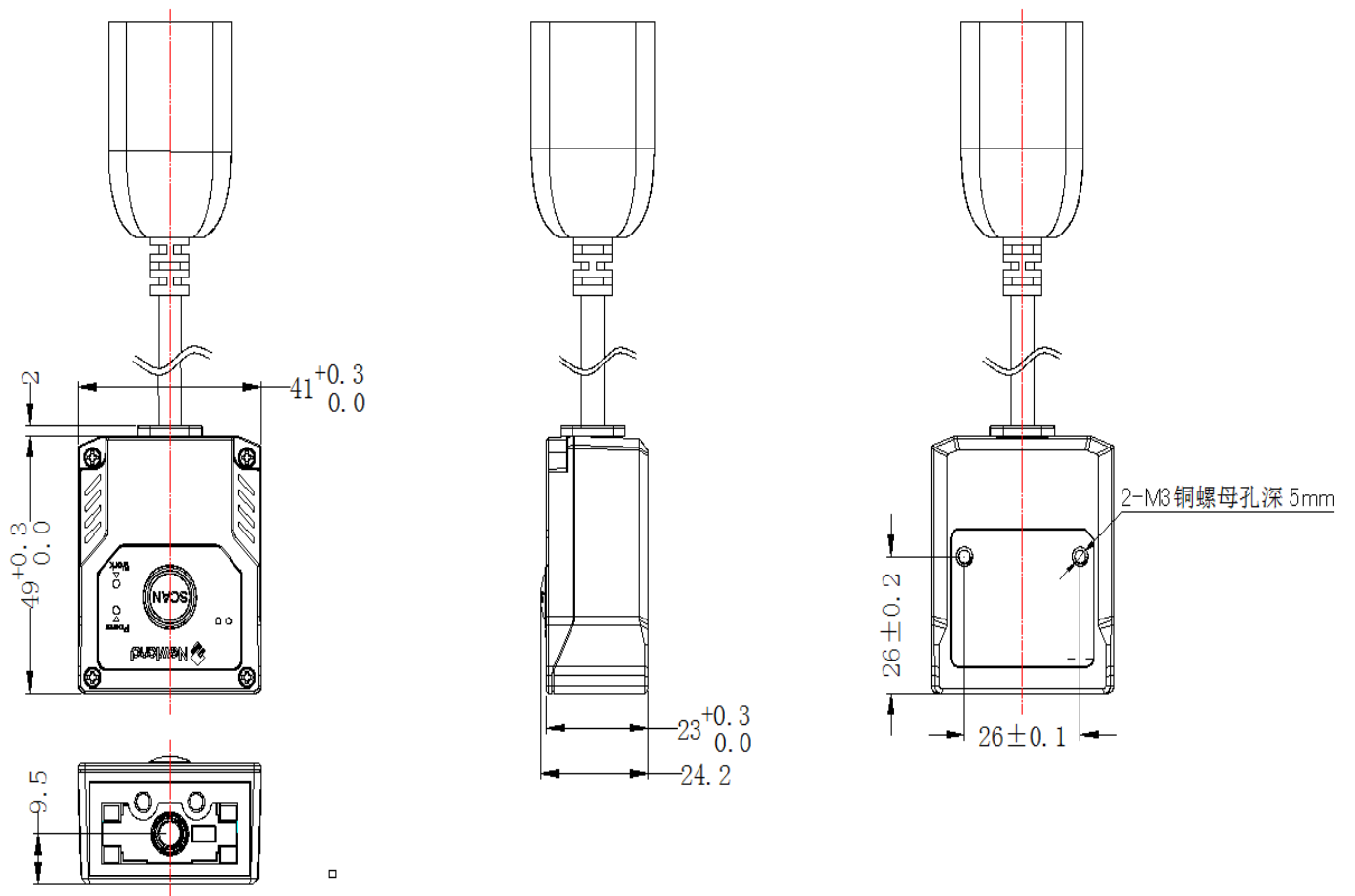
三视图
