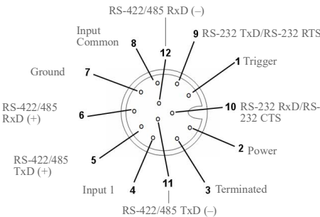
连接器 B( 串行型号 ) M12 12 引脚插座
