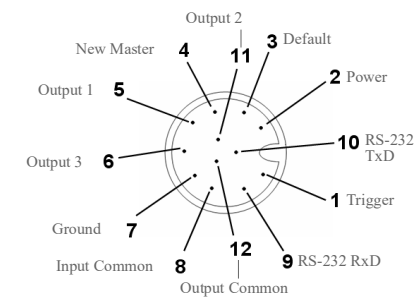
连接器 A( 所有型号 ) 的 M12 12 引脚插头
