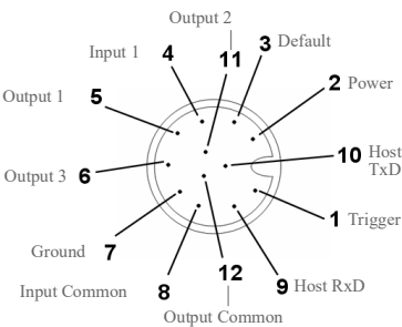
连接器 A( 所有型号 ) M12 12 引脚插头
